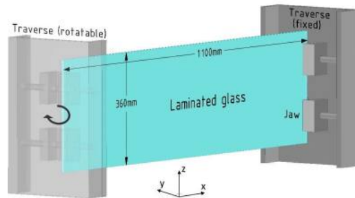
Abb. A 4.2: Torsionsrelaxationsversuch
